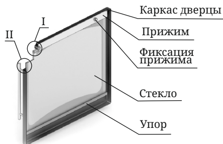
Рисунок 6. Ремонт светопрозрачного экрана дверцы «Люмина»
