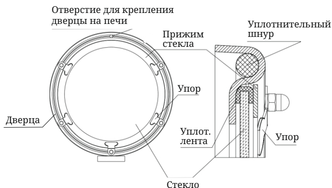
Рисунок 8. Ремонт светопрозрачного экрана (стекла) иллюминатора
