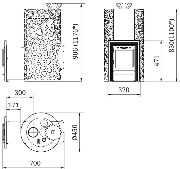
Рисунок 1. Габаритно-монтажные размеры печей «Аврора», «Аврора Макси»
