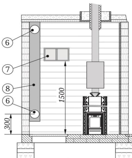
Рисунок 3. Схема монтажа печи
