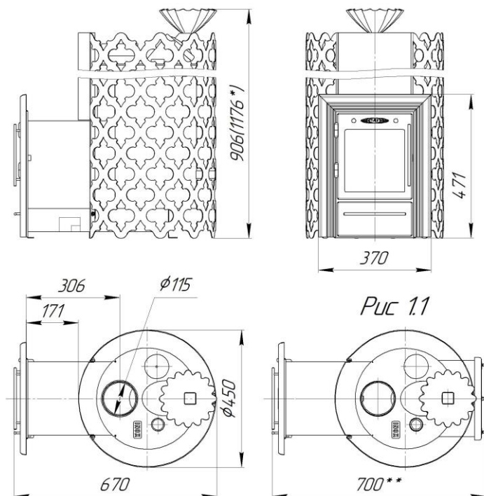
Рисунок 1. Габаритно-монтажные размеры печей «Арабеска Люмина», «Арабеска Супер Inox» и «Арабеска Макси Люмина»*
