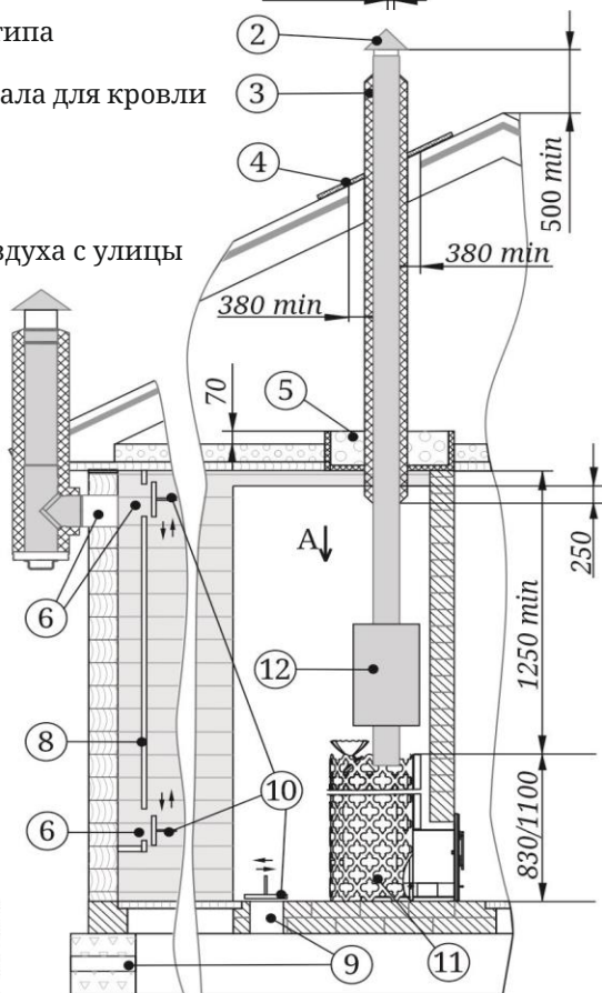
Рисунок 3. Схема монтажа печи
