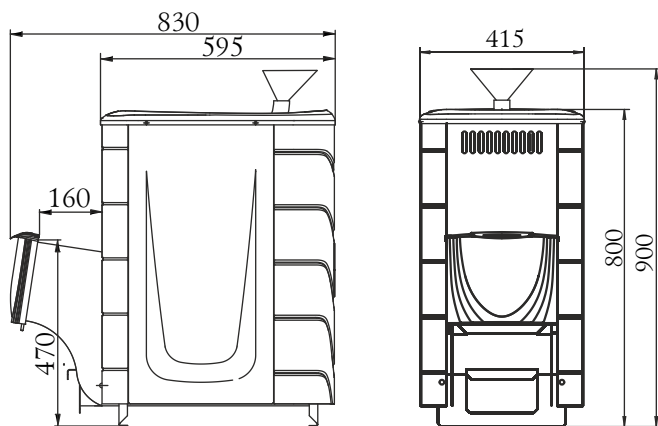
Рисунок 1. Габаритные размеры печи «Ангара 2012 Inox» и «Ангара 2012 Carbon».
