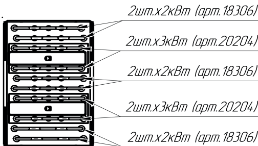
Рис. 1.3 Распределения ТЭНов по кол-ву и мощности 24-72 кВт
