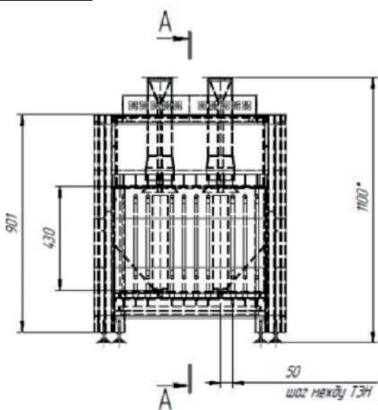
Рис. 1.2.1 Внешний вид Устройства при односекционном исполнении
