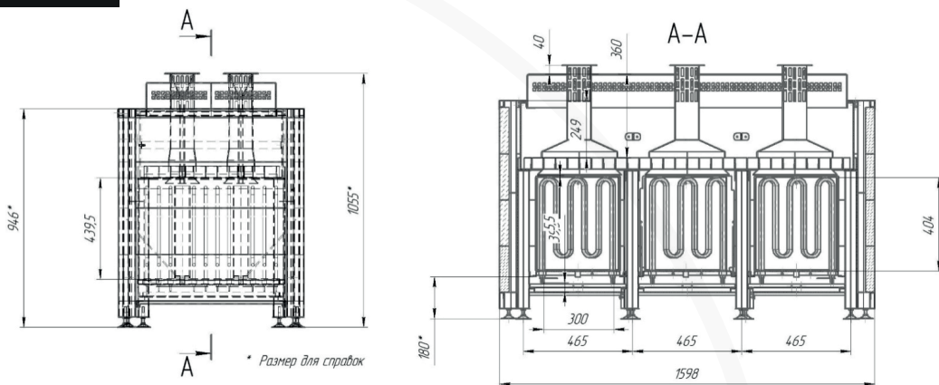
Рис. 1.2.3 Внешний вид Устройства при трехсекционном исполнении
