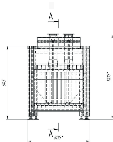
Рис. 1.2.2 Внешний вид Устройства при двухсекционном исполнении
