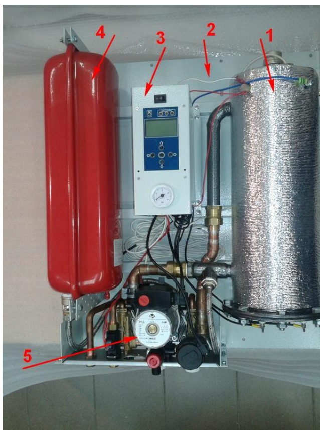
Рисунок 2. Общий вид водонагревателя «Premium»
