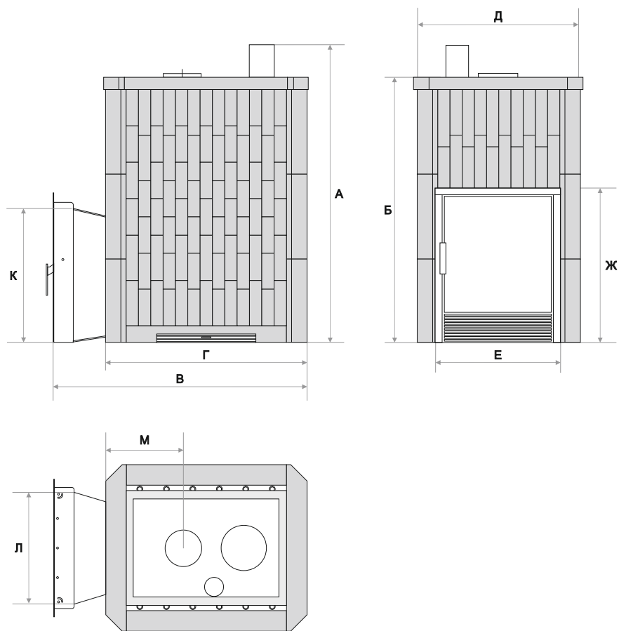
Рис. 21 Габаритные размеры печи
