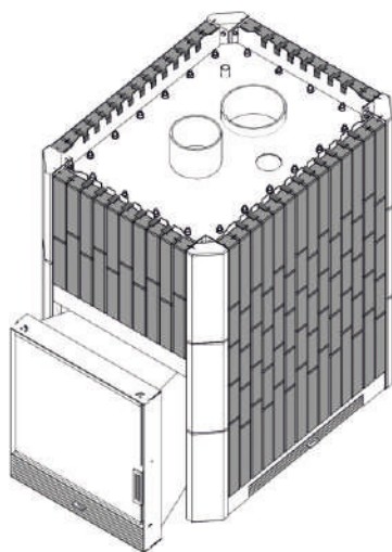
Рис. 17 Установка боковых ламелей
