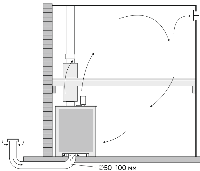
Рис. 6 Естественная вентиляция
