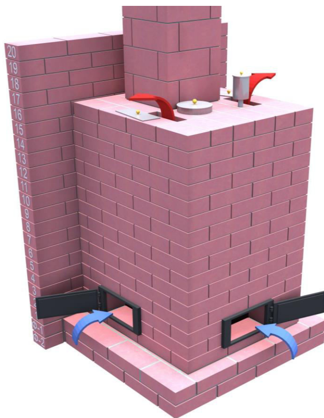
Рис. 9 Пример перекрытия верха печи кирпичем
