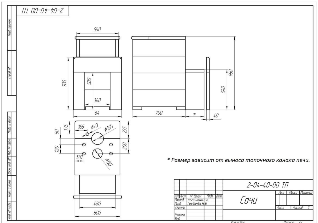
Рис. 14 Размеры экрана из природного камня (талькохлорита)
