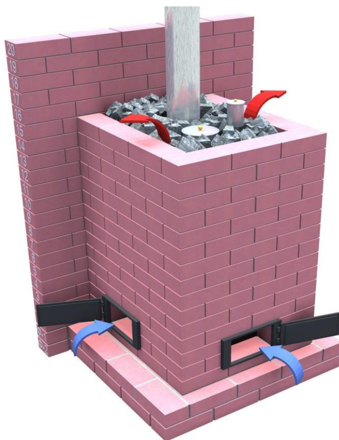
Рис. 7 Пример декорирования верха печи камнями
