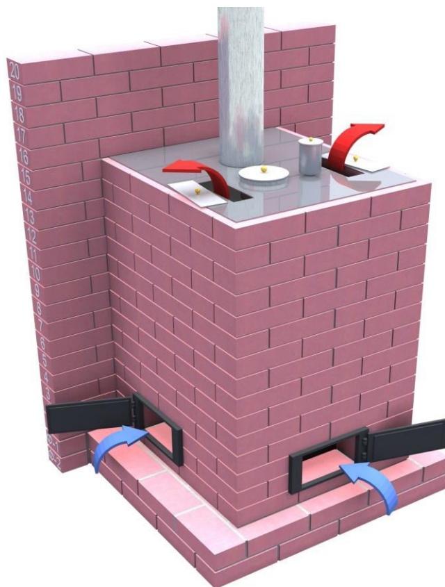
Рис. 11 Внешний вид печи с листом перекрытия
