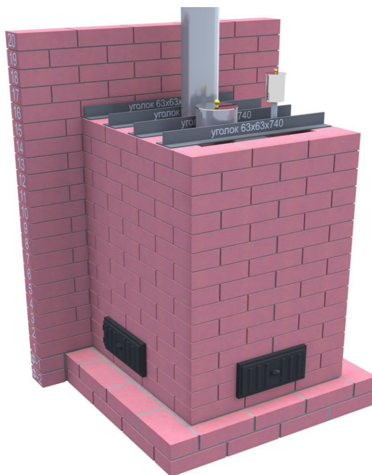
Рис. 8 Установка вспомогательных уголков
